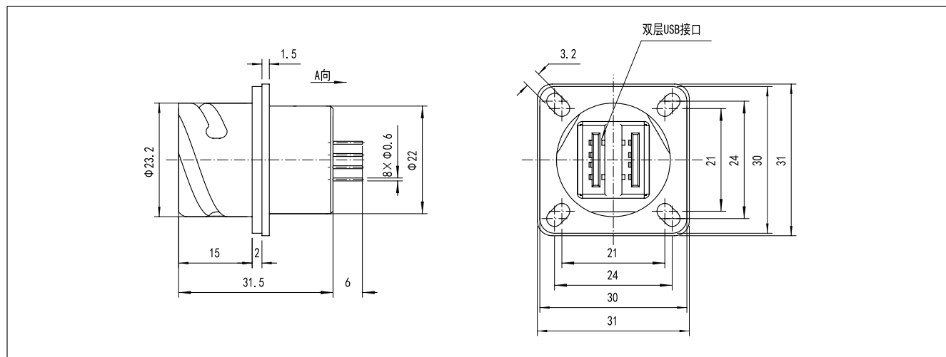
推荐面板开孔尺寸
