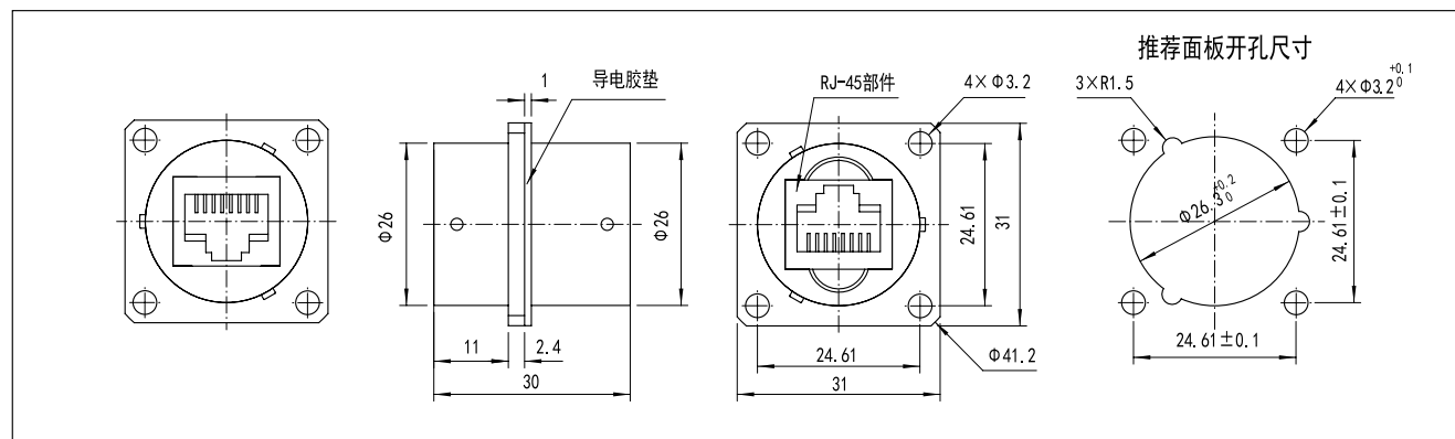
[CT55E-8Z-01 双卡口连接法兰安装转接插座]
