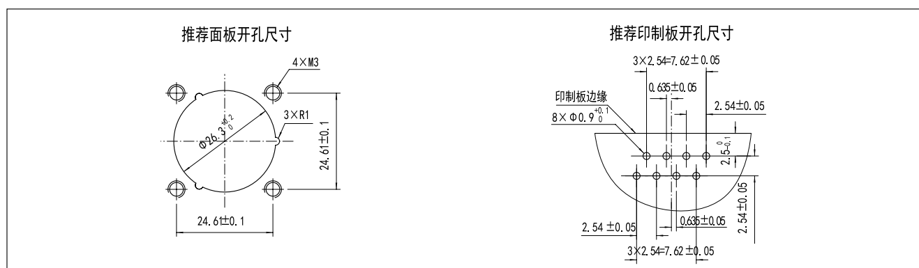
[CT55E-8Z 单卡口连接法兰安装转接插座]
