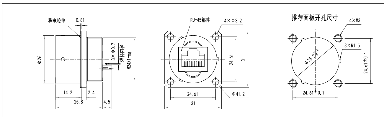
[CT55-8ZS-03 方盘安装插座, 尾部焊线杯焊线]
