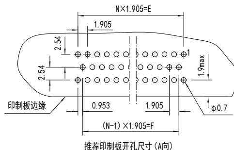
推荐印制板开孔尺寸(A向)
