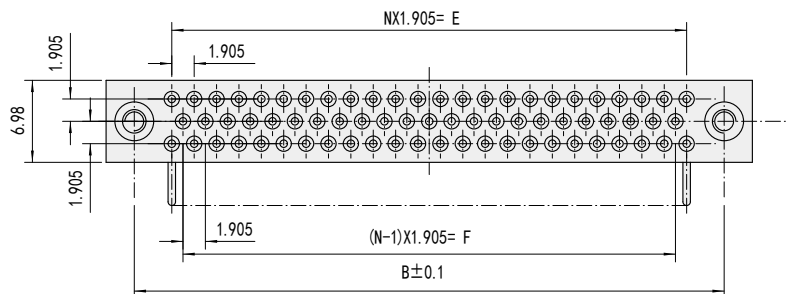
直插型安装紧固件示意: 5500
