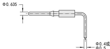
31 插针，弯式浸焊，引脚长度2.77mm，直径 \Phi 0.5
