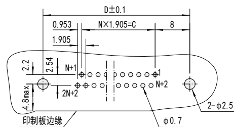
推荐印制板开孔尺寸(A向)
