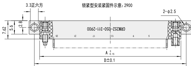
锁紧型安装紧固件示意: 2900
