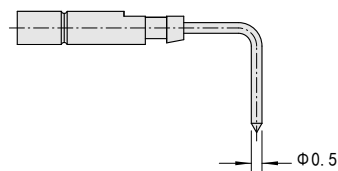
44 插孔，弯式浸焊，引脚长度2.77mm
