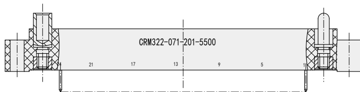
直插型安装紧固件示意: 5500
