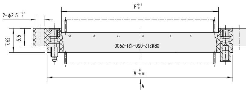
锁紧型安装紧固件示意: 2900
