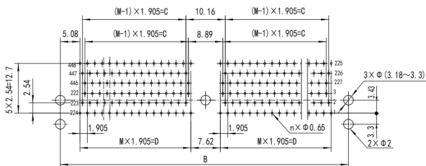
推荐印制板开孔尺寸图(F向)
