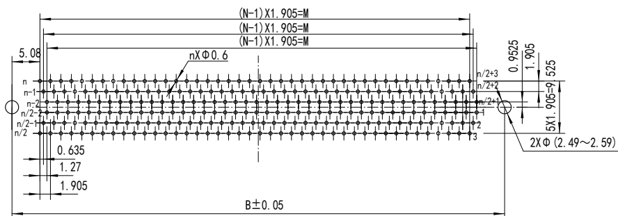
推荐印制板开孔尺寸图 (F向)
