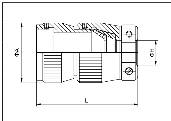
【屏蔽式电缆罩 Y11X-XX00-86】
