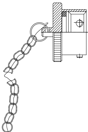
【热缩套管式1型电缆罩 Y11X-XX00-84】
