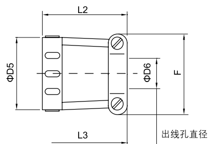
直式电缆夹
