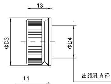
屏蔽螺帽
