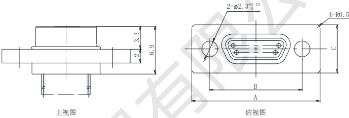
产品外形尺寸图
