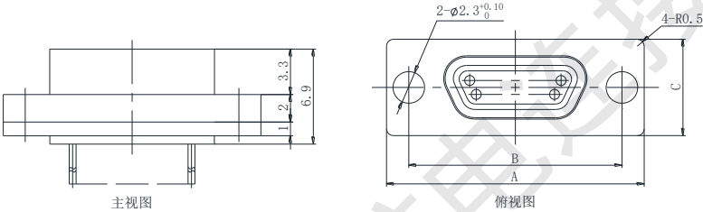
产品外形尺寸图
