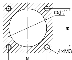
YMC插座面板开孔尺寸
