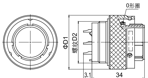
插头YMC-TB-P(焊接接触件)
