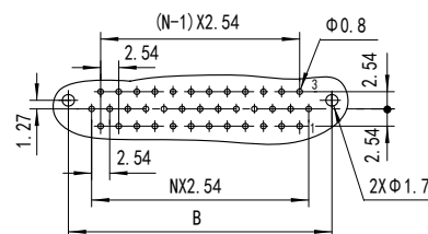
CY23Z-BJ-DL推荐印制板开孔尺寸 (E向) 3排
