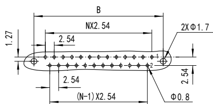
CY23Z-BJ-DL推荐印制板开孔尺寸 (E向) 2排
