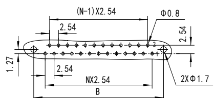
CY23Z-BJ-DL推荐印制板开孔尺寸 (E向) 2排
