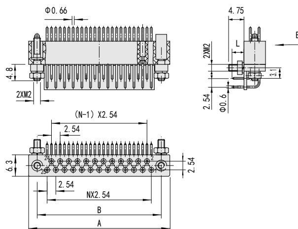
弯式插座（装针）
