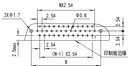
CY23T-WJ-DW推荐印制板开孔尺寸 (E向) 3排
