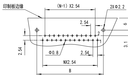
CY23P-WJ-RL推荐印制板开孔尺寸（E向）
