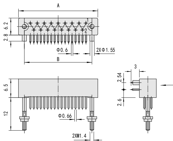
插座 CY23P-WJ-GL
