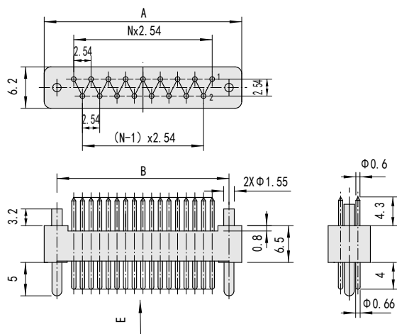
直式插头
