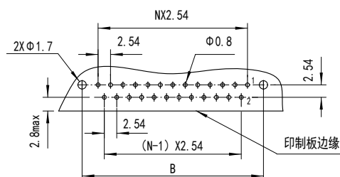
CY23P-WJ-GL推荐印制板开孔尺寸 (E向)
