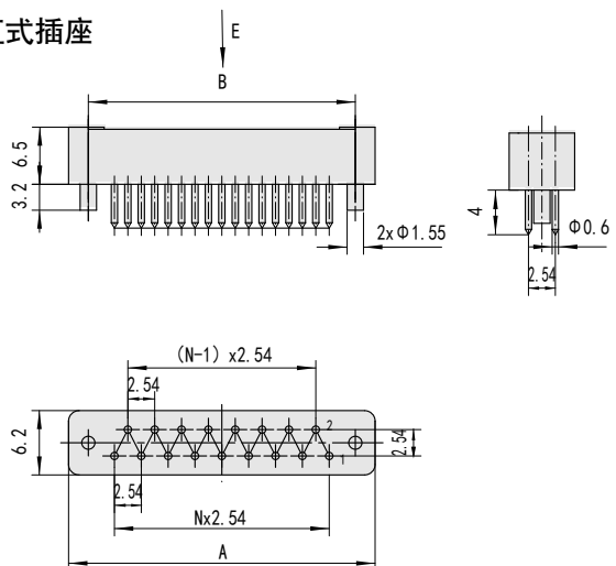
直式焊接插座
