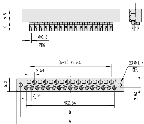
自由插头 CY23S-HJ
