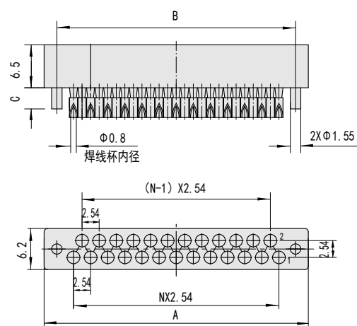
直式焊接插座
