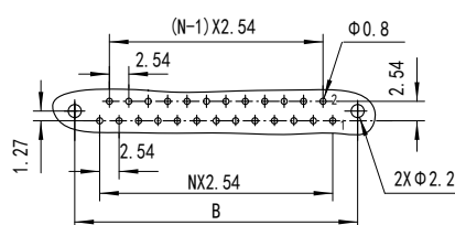
CY23P-BJ-RL推荐印制板开孔尺寸（E向）
