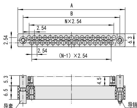
自由插头（装孔）
