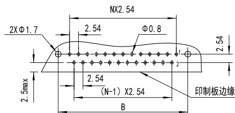
CY23T-WJ-DW推荐印制板开孔尺寸 (E向) 2排
