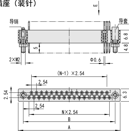
直式插座（装针）
